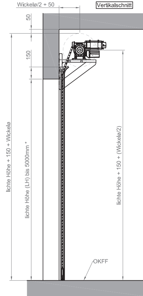
Vertikalschnitt
