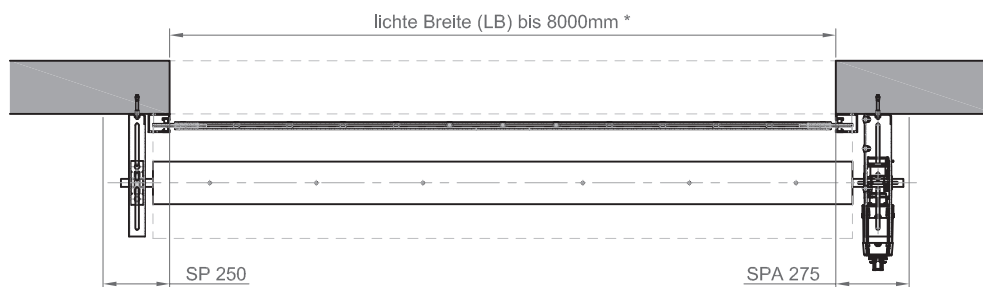
Horizontalschnitt
